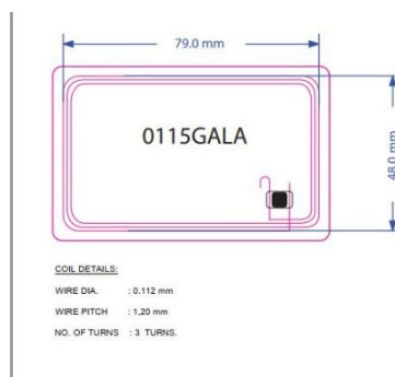
0115GALA Antenna
